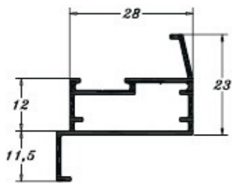
PE 0550 0,331 Kg/m
