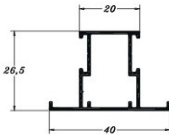
PE 0556 0,351 Kg/m
