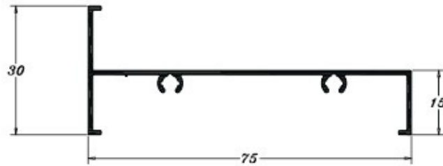
PE 0544 0,383 Kg/m
