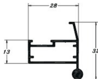
PE 0553 0,363 Kg/m
