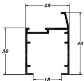
PE 0552 0,333 Kg/m
