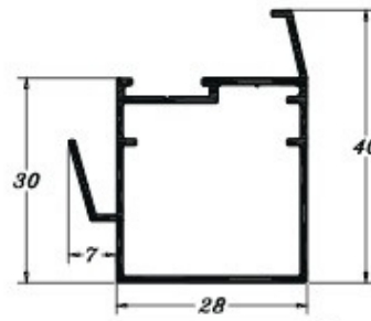
PE 0547 0,412 Kg/m
