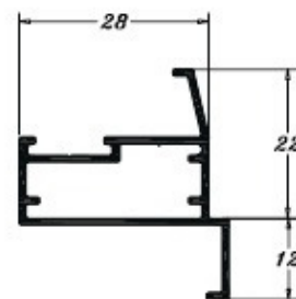
PE 0551 0,323 Kg/m
