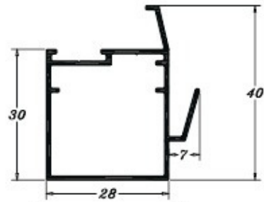
PE 0548 0,412 Kg/m
