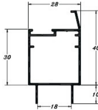
PE 0549 0,425 Kg/m
