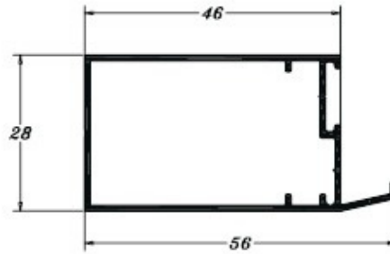
PE 0555 0,457 Kg/m
