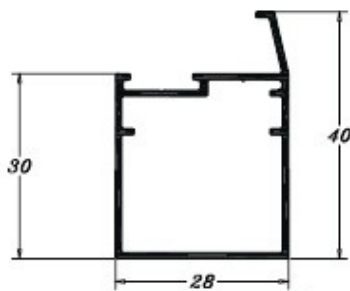
PE 0546 0,371 Kg/m
