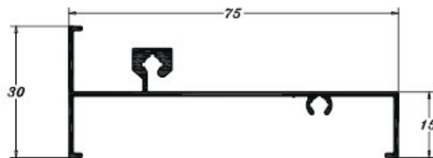
PE 0558 0,478 Kg/m
