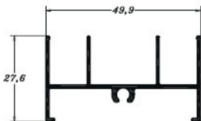
PE0775 0,445 Kg/m
