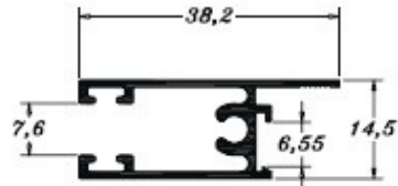
PE0772 0,319 Kg/m
