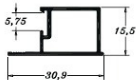
PE0773 0,217 Kg/m
