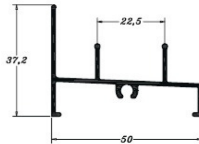
PE0774 0,450 Kg/m
