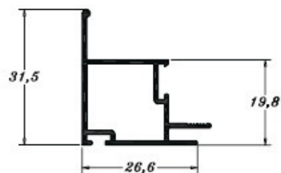
PE0776 0,297 Kg/m
