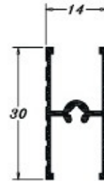
I 154 0,230 Kg/m
