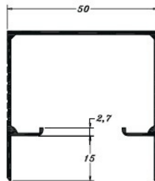
U 655 0,555 Kg/m
