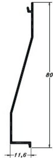
PE 0338 0,267 Kg/m
