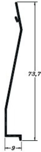
PE 0053 0,233 Kg/m
