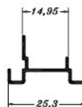
PE0314 0,132 Kg/m
