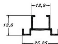
PE0347 0,149 Kg/m
