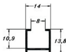
PE0313 0,112 Kg/m
