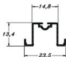
PE0662 0,134 Kg/m
