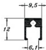
PE0782 0,128 Kg/m
