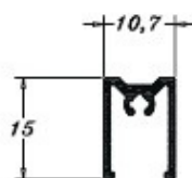
PE0346 0,128 Kg/m
