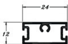
PE0315 0,248 Kg/m
