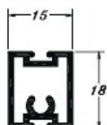
PE0054 0,275 Kg/m
