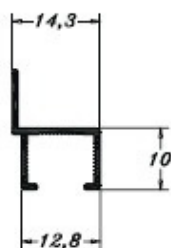
PE0345 0,113 Kg/m
