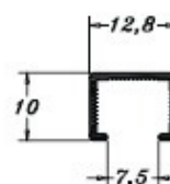
PE0344 0,084 Kg/m
