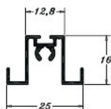
PE0860 0,213 Kg/m
