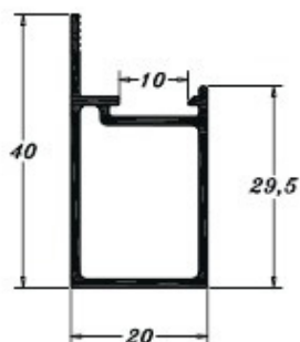
PE0867 (MP300) 0,387 Kg/m
