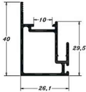
PE0869 (MP302) 0,474 Kg/m
