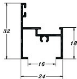
PE0855 (MP312) 0,270 Kg/m
