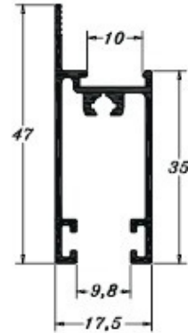
PE0870 (MP309) 0,396 Kg/m
