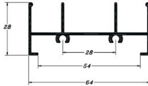
PE0864 (MP357) 0,642 Kg/m
