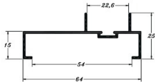
PE0866 (MP360) 0,441 Kg/m
