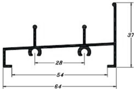
PE0865 (MP358) 0,605 Kg/m
