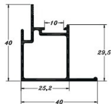
PE0868 (MP321) 0,498 Kg/m
