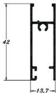
PE 0280 0,295 Kg/m
