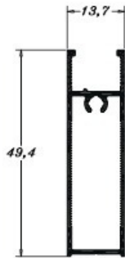
PE 0277 0,335 Kg/m
