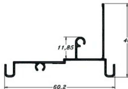
PE 0281 0,380 Kg/m
