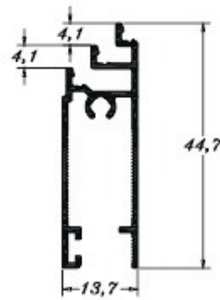
PE 0278 0,325 Kg/m
