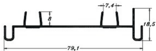
PE 0285 0,391 Kg/m
