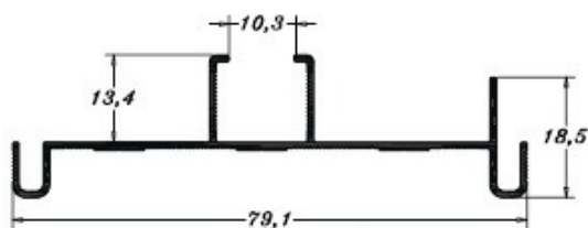
PE 0286 0,390 Kg/m
