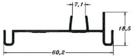
PE 0282 0,306 Kg/m
