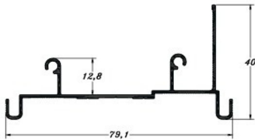
PE 0284 0,467 Kg/m
