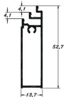
PE 0279 0,369 Kg/m
