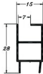
PE0484 0,217 Kg/m
