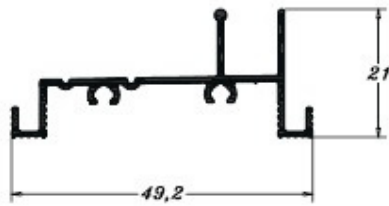
PE0525 0,309 Kg/m
