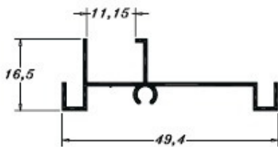
PE0617 0,225 Kg/m
