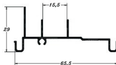
PE0524 0,378 Kg/m
