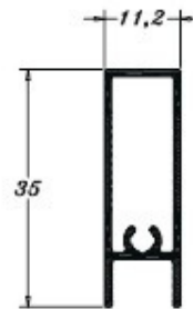
PE0522 0,255 Kg/m
