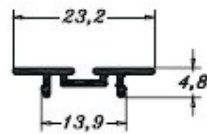
PE0571 0,102 Kg/m
