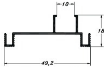
PE0526 0,260 Kg/m
