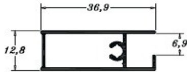
PE0490 0,275 Kg/m
