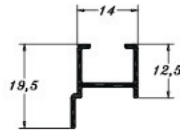
PE0365 0,132 Kg/m
