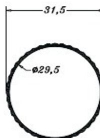
PE 0033 0,223 Kg/m
