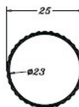
PE 0200 0,173 Kg/m
