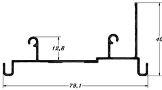
PE 0284 0,467 Kg/m
