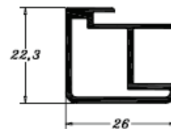
PE 0391 0,380 Kg/m
