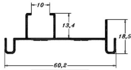
PE 0283 0,336 Kg/m
