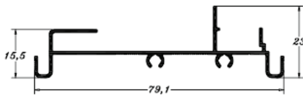
PE 0319 0,440 Kg/m
