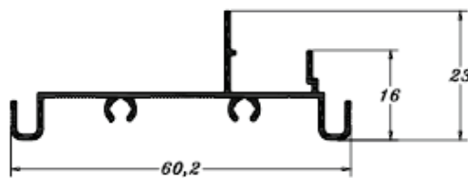
PE 0321 0,332 Kg/m
