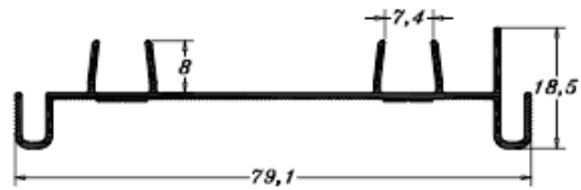
PE 0285 0,391 Kg/m
