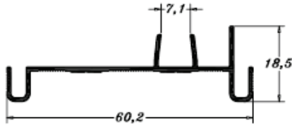
PE 0282 0,306 Kg/m
