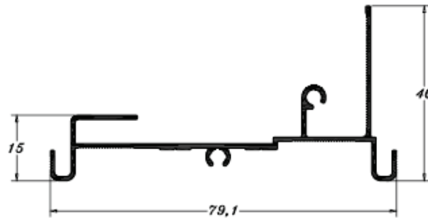
PE 0316 0,496 Kg/m
