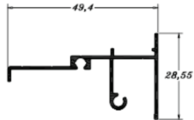
PE 0320 0,325 Kg/m
