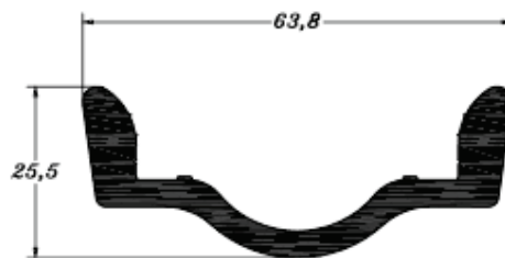
PE 0454 1,191 Kg/m
