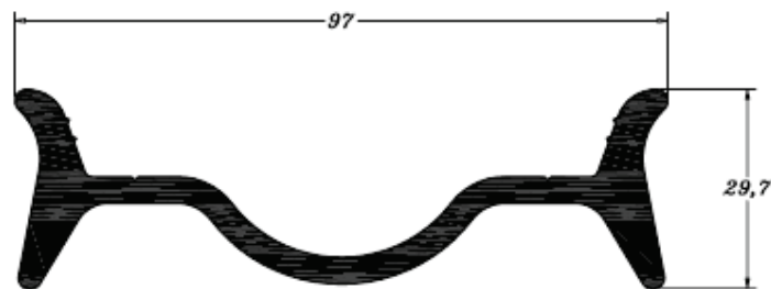
PE 0612 1,870 Kg/m
