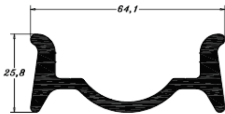
PE 0452 1,289 Kg/m
