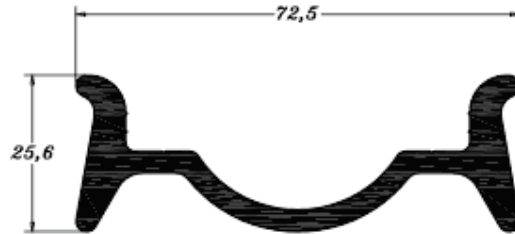
PE 0453 1,378 Kg/m
