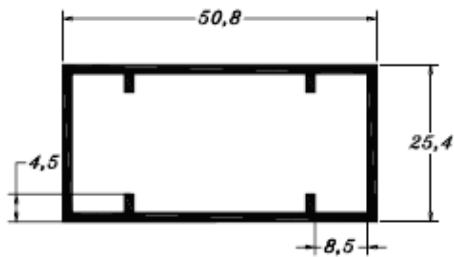
D 079 0,643 Kg/m
