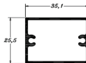
D055 0,479 Kg/m
