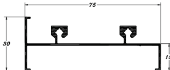
PE 0557 0,574 Kg/m
