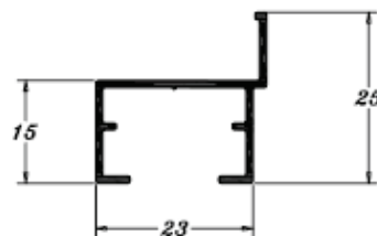
PE 0543 0,196 Kg/m
