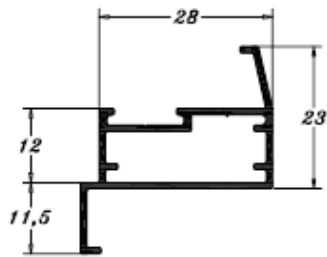
PE 0550 0,331 Kg/m
