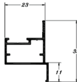
PE 0542 0,292 Kg/m
