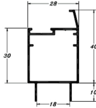
PE 0549 0,425 Kg/m
