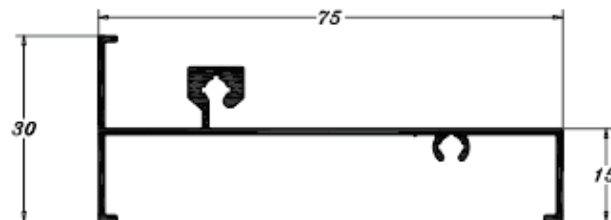
PE 0558 0,478 Kg/m
