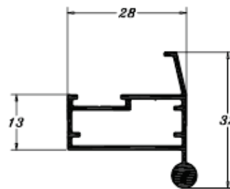
PE 0553 0,363 Kg/m
