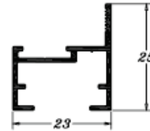
PE 0540 0,222 Kg/m
