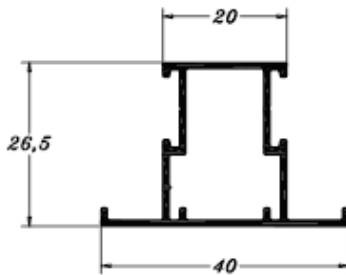
PE 0556 0,351 Kg/m
