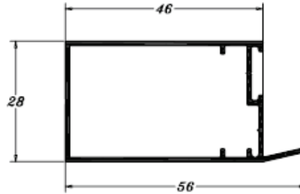
PE 0555 0,457 Kg/m
