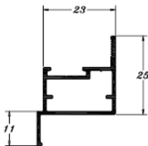
PE 0541 0,292 Kg/m
