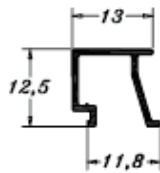
PE 0554 0,100 Kg/m
