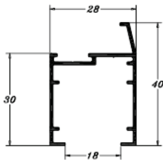
PE 0552 0,333 Kg/m
