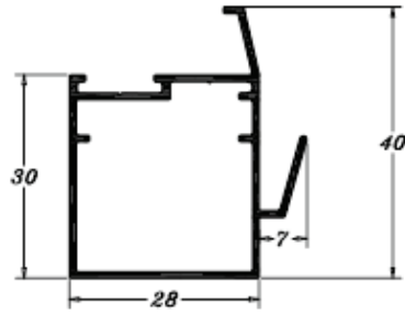
PE 0548 0,412 Kg/m
