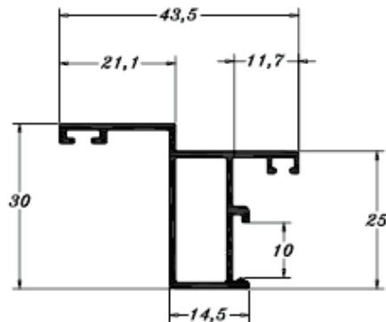
P146 0,391 Kg/m
