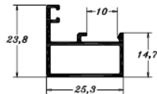
P147 0,298 Kg/m
