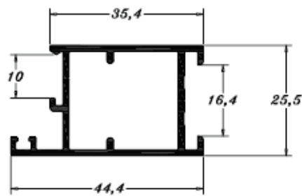
P416 0,564 Kg/m
