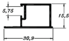
PE0773 0,217 Kg/m
