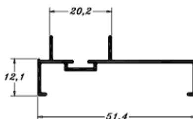
PE0783 0,274 Kg/m
