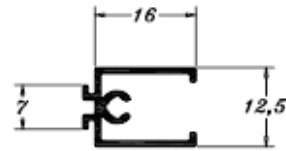
PE0261 0,154 Kg/m
