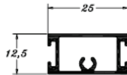
PE0262 0,252 Kg/m
