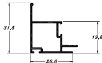
PE0776 0,297 Kg/m
