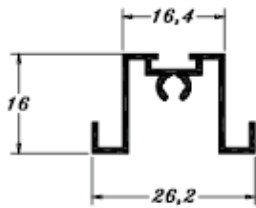
PE0059 0,198 Kg/m
