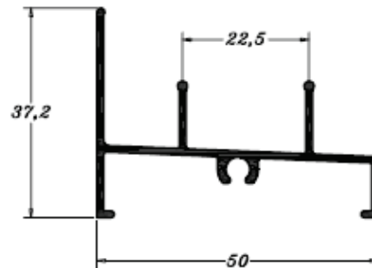
PE0774 0,450 Kg/m
