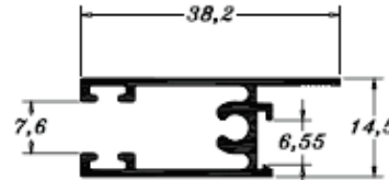
PE0772 0,319 Kg/m
