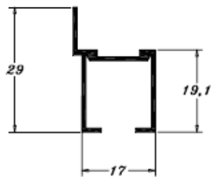
PE0265 0,197 Kg/m
