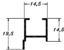
PE0181 0,127 Kg/m
