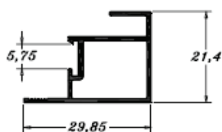
PE0777 0,254 Kg/m
